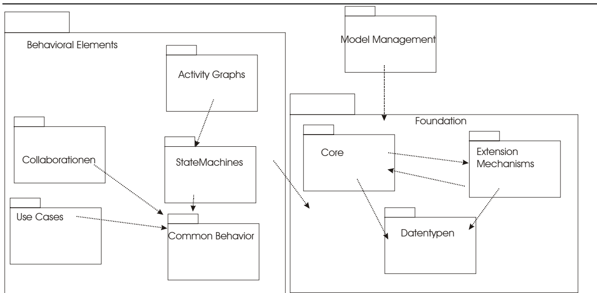
Abbildung 1-2; Das UML- Metamodell
